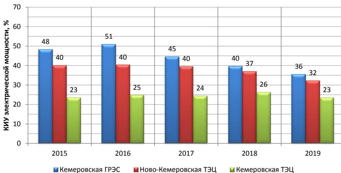
Рисунок 2-11 – Средний по электростанциям ООО «СГК» коэффициент использования установленной электрической мощности
