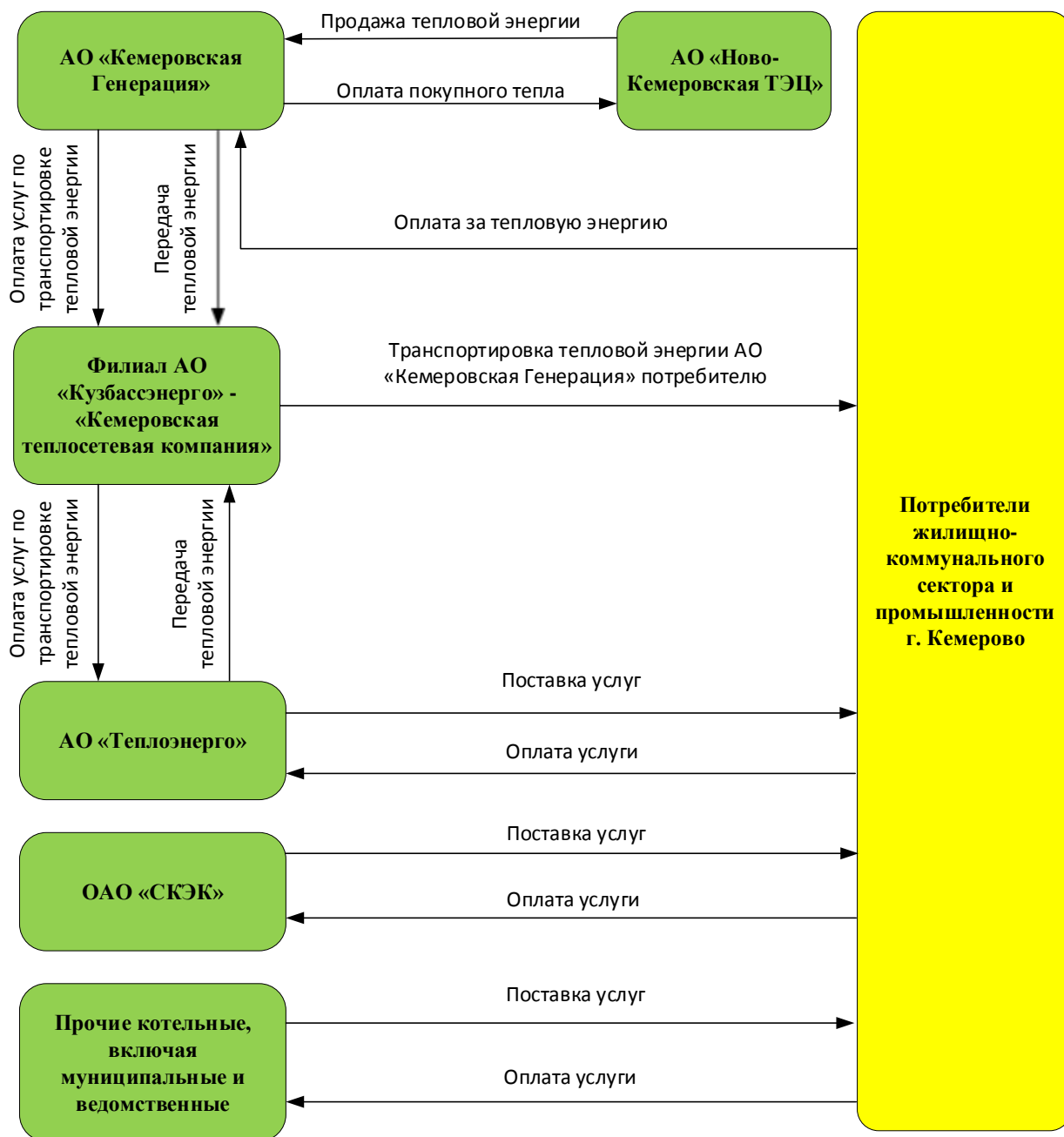
Рисунок 1-1 – Функциональная структура системы теплоснабжения г. Кемерово
