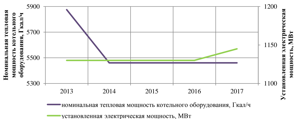
Рисунок 2-1 – Распределение установленной тепловой и электрической мощности источников ООО «СГК» по годам
