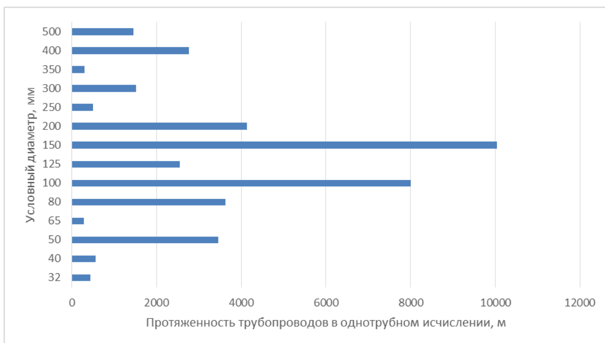
Рисунок 3.17 – Распределение протяженности тепловых сетей ОАО «СКЭК» по диаметрам трубопроводов.
