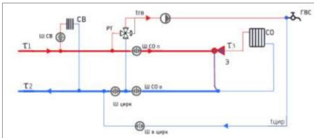
Рисунок 3.13 – Потребитель с открытым водоразбором на ГВС и элеваторным присоединением СО (схема № 6)
